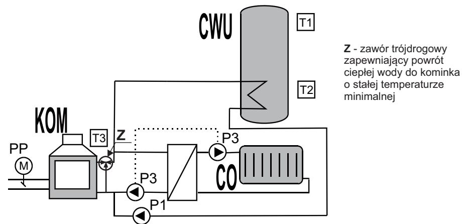
Rys.1b Układ pracy regulatora z wymiennikiem dla obwodu CO (pompa wymiennika i CO podłączone do wyjścia P3)
